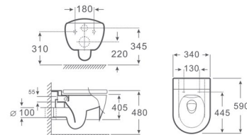
DG143 直冲式挂墙坐便器 Washdown Wall-hung Toilet Size: 590x340x405mm P-trap, 180mm Roughing-in 横排污口中心离地180mm
