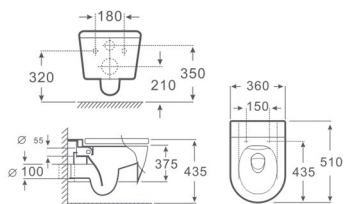
DG167 直冲式挂墙坐便器 Washdown Wall-hung Toilet Size: 510x360x375mm P-trap, 180mm Roughing-in 横排污口中心离地180mm
