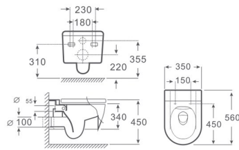
DG115 直冲式挂墙坐便器 Washdown Wall-hung Toilet Size:560x350x340mm P-trap,180mm Roughing-in 横排污口中心离地180mm
