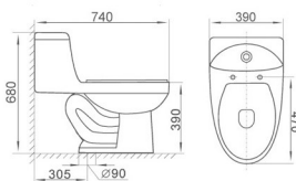
DA8008 虹吸连体坐便器 Siphonic One-piece Toilet Size:740x390x680mm S-trap,305mm Roughing-in 地排污口中心离墙305mm
