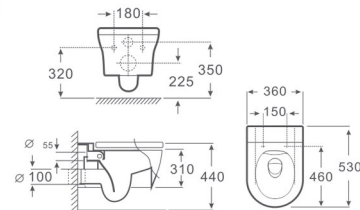
超漩 DG177 超漩式挂墙坐便器 Eddy double hole Wall-hung Toilet Size: 530x360x310mm P-trap, 180mm Roughing-in 横排污口中心离地180mm
