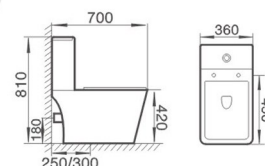
DA8030 直冲连体坐便器 Washdown One-piece Toilet Size:700x360x810mm S-trap,250mm Roughing-in 地排污口中心离墙250mm P-trap,180mm Roughing-in 横排污口中心离地180mm
