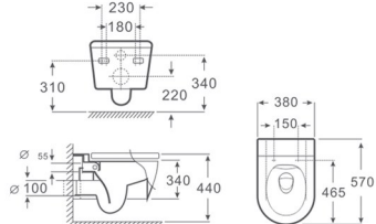
DG111 直冲式挂墙坐便器 Washdown Wall-hung Toilet Size: 570x380x340mm P-trap, 180mm Roughing-in 横排污口中心离地180mm
