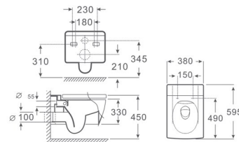
DG113 直冲式挂墙坐便器 Washdown Wall-hung Toilet Size: 595x380x330mm P-trap, 180mm Roughing-in 横排污口中心离地180mm
