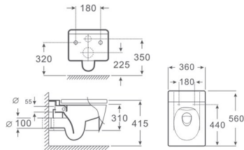
DG133 直冲式挂墙坐便器 Washdown Wall-hung Toilet Size:560x360x310mm P-trap,180mm Roughing-in 横排污口中心离地180mm
