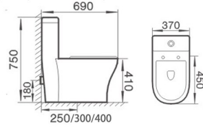
DA8070 虹吸/直冲连体坐便器 Siphonic/Washdown One-piece Toilet Size: 690x370x750mm S-trap, 250, 300, 400mm Roughing-in 地排污口中心离墙250, 300, 400mm P-trap, 180mm Roughing-in 横排污口中心离地180mm
