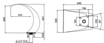
眼镜蛇瀑布 Model No:M02
