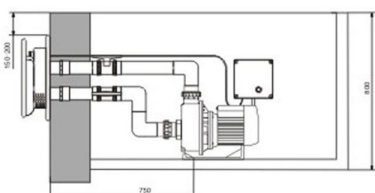
Swim jet MC2000型
