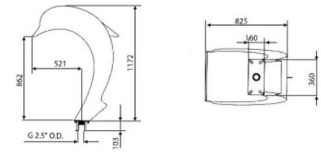
海豚瀑布 Model No:M03
