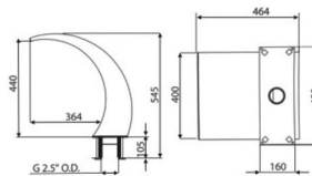
朗多瀑布 Model No:M05
