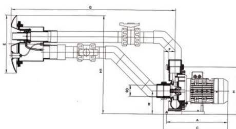
Swim jet MC1000型
