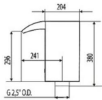
梯级瀑布 Model No:M04
