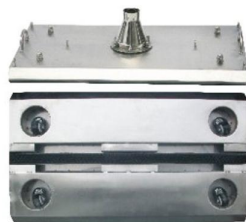
吸污盘 700x400mm Model No:M08
