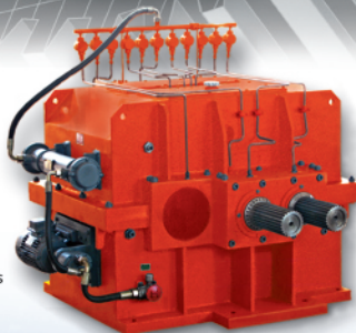
● AF系列齿轮 减速电动机 Series AF Geared Motors
