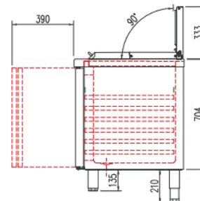
MFE-200
