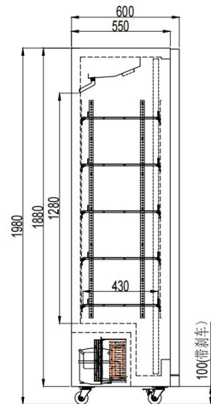
闭门侧视图
