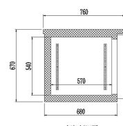
门侧视图
