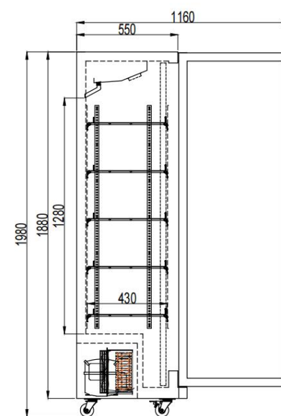
开门侧视图
