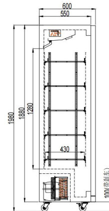
闭门侧视图
