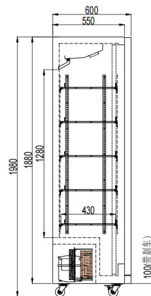
闭门侧视图
