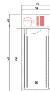
开门侧视图
