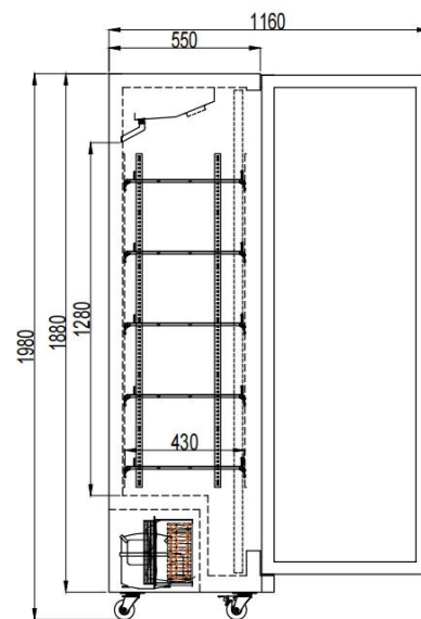
开门侧视图
