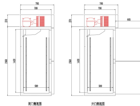
闭门侧视图
