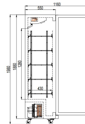
开门侧视图
