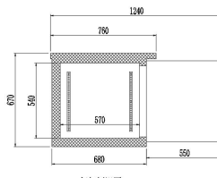
门前视图
