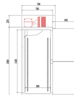
开门侧视图
