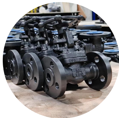
美标法兰闸阀 Z41H-150LB
