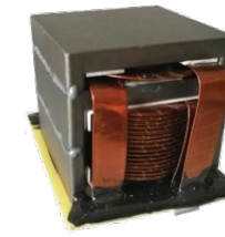
■ 扁平立绕变压器 Flat Wire Vertical Wound Transformer
