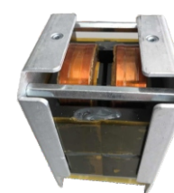
■ 扁平立绕变压器 Flat Wire Vertical Wound Transformer
