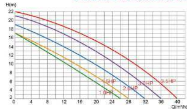
性能曲线图 Performance chart
