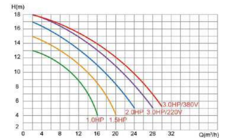
性能曲线图 Performance chart
